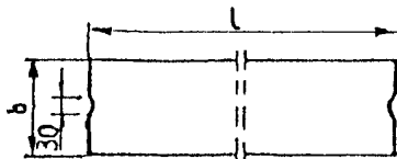
Rys. 1. Wymiarowanie krawężników
